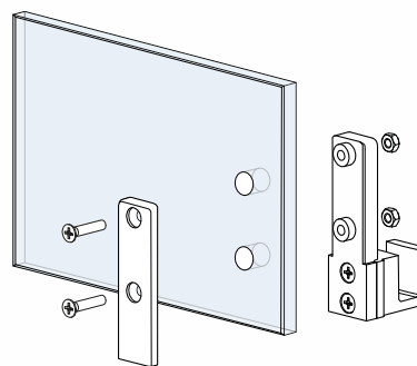
Montážní schéma dolního profilu Bottom track installation scheme
