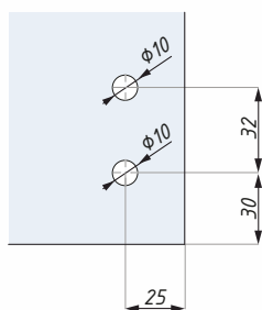
Příprava skla pro dolní profil Glass preparation for bottom track
